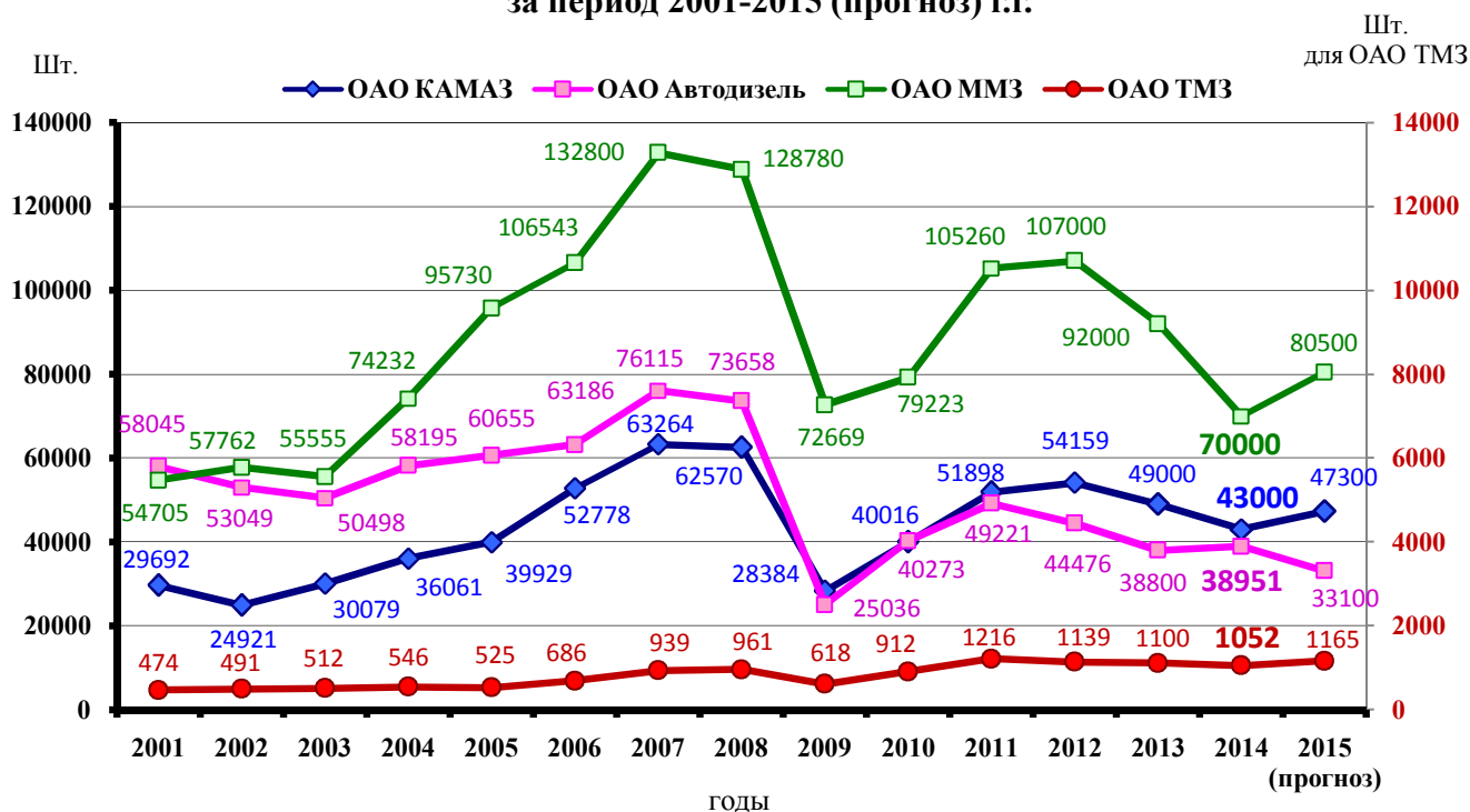
Динамика производства автотракторных дизельных двигателей за период 2001-2015 (прогноз) г.г.
