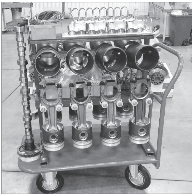
Тележка с деталями для сборки двигателя
