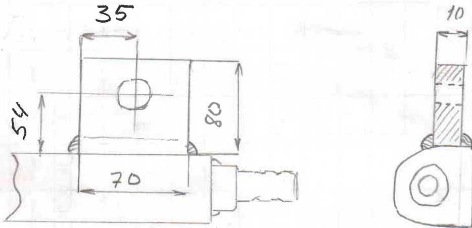
ПЛОЩАДКА СОЕДИНИТЕЛЬНАЯ 70 (перемычка)
