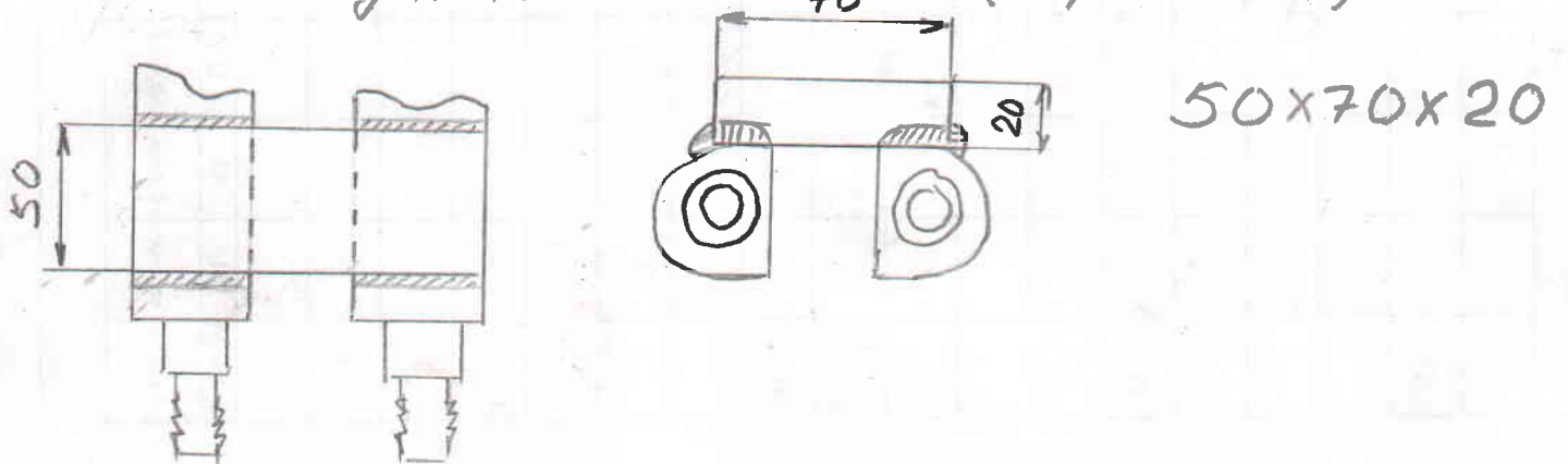
ПЛОЩАДКА СОЕДИНИТЕЛЬНАЯ 70 (перемычка)
